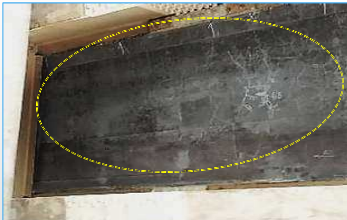
亀甲状クラック+エフロ
