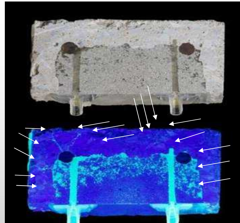
断面修復後注入確認実験
