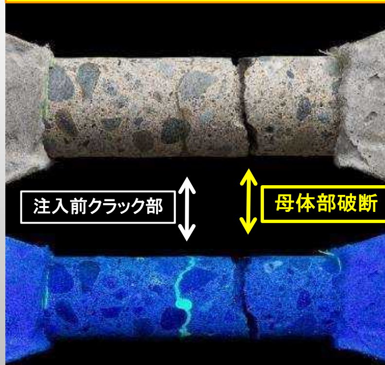
岐阜大学 注入後の引張試験
