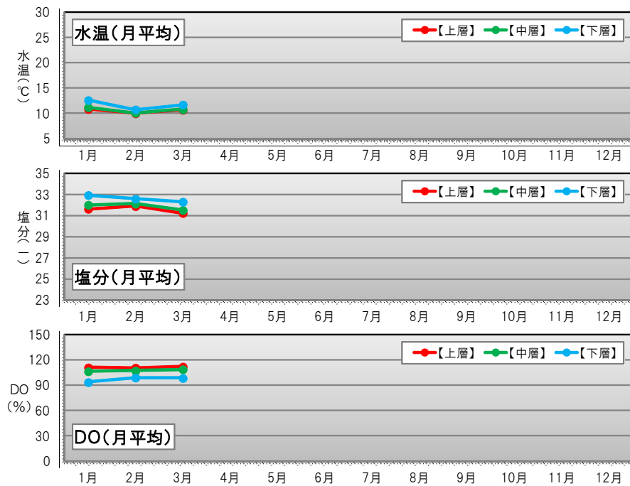
図 4-1(3) 月平均値の変化(川崎人工島)
