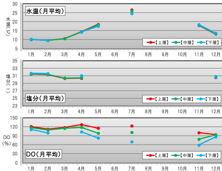
図4-1(1) 月平均値の変化(千葉港港波浪観測塔)
