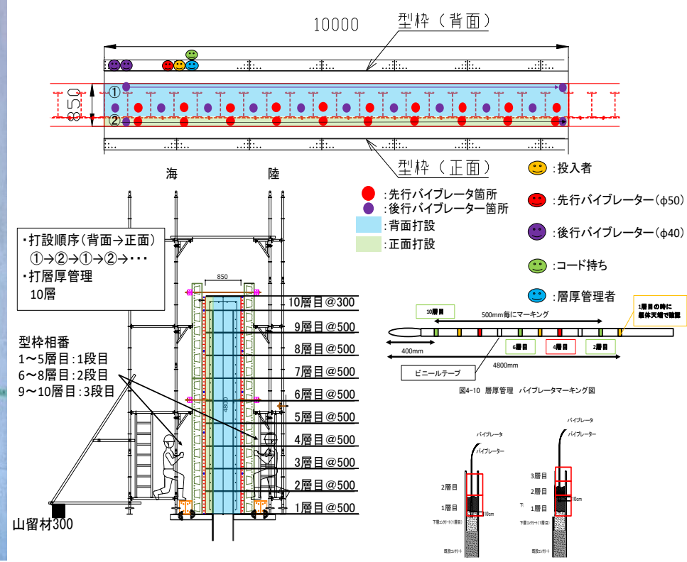
打設手順書 (一部抜粋)
