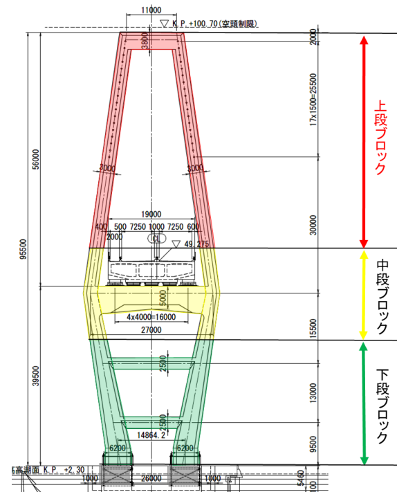
主塔正面図
