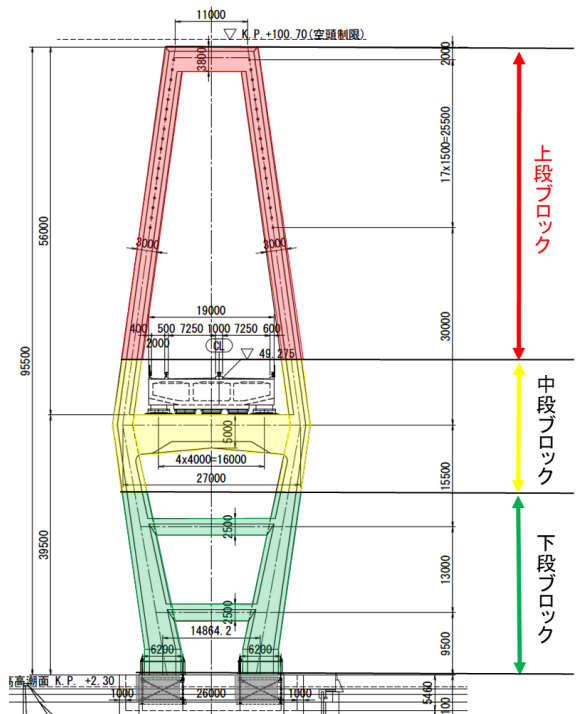
主塔正面図
