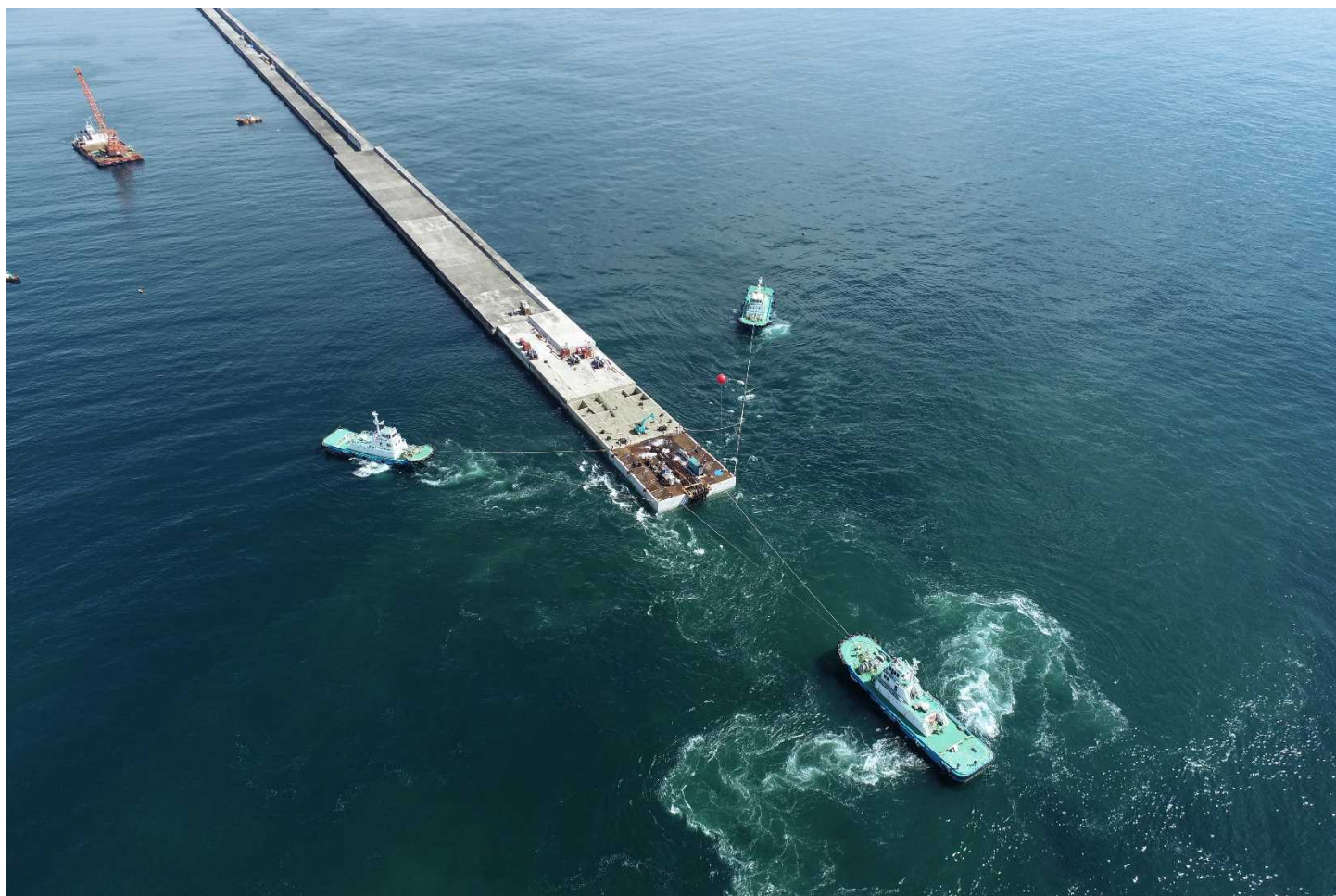
茨城港常陸那珂港区外港地区東防波堤 ケーソン据付
