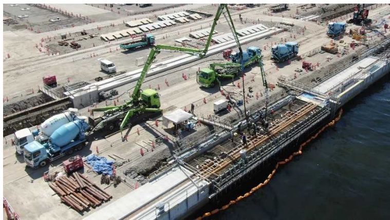
横浜港本牧地区岸壁(-16m) 岸壁上部コンクリート打設、若手職員安全確認
