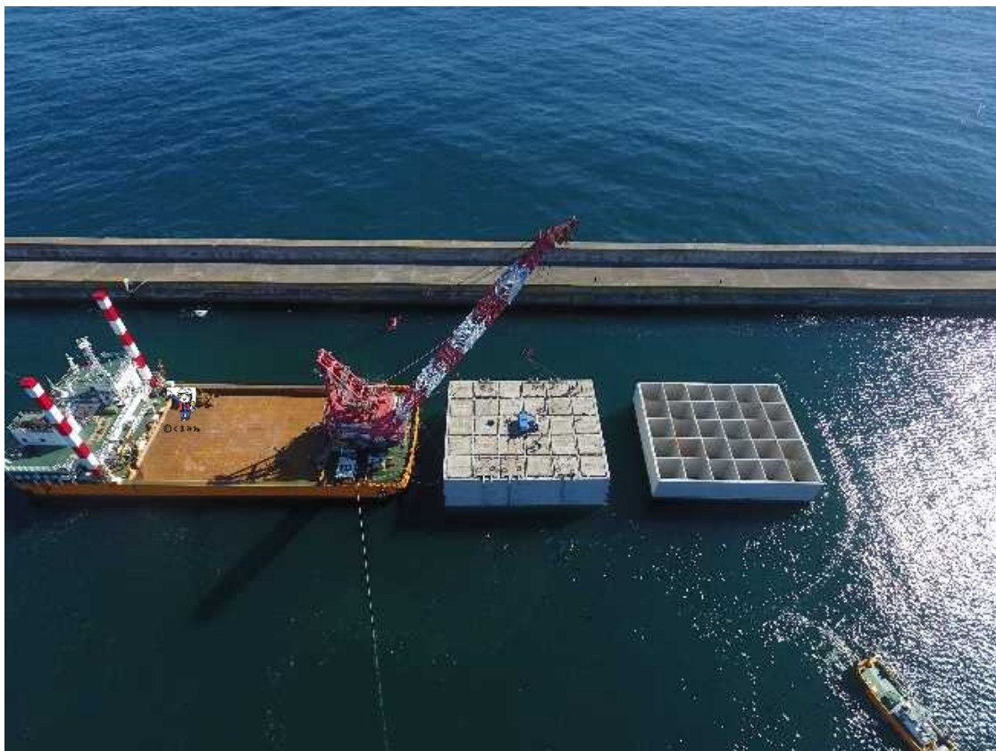
常陸那珂港区外港地区東防波堤 ケーソン仮置き
