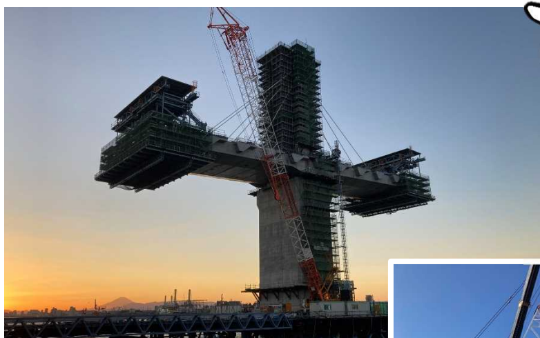
川崎港臨港道路 主橋梁上部 (MP2)
