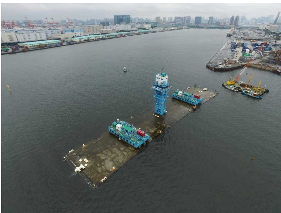
(右) 沈埋箱(最終箱) 沈設
