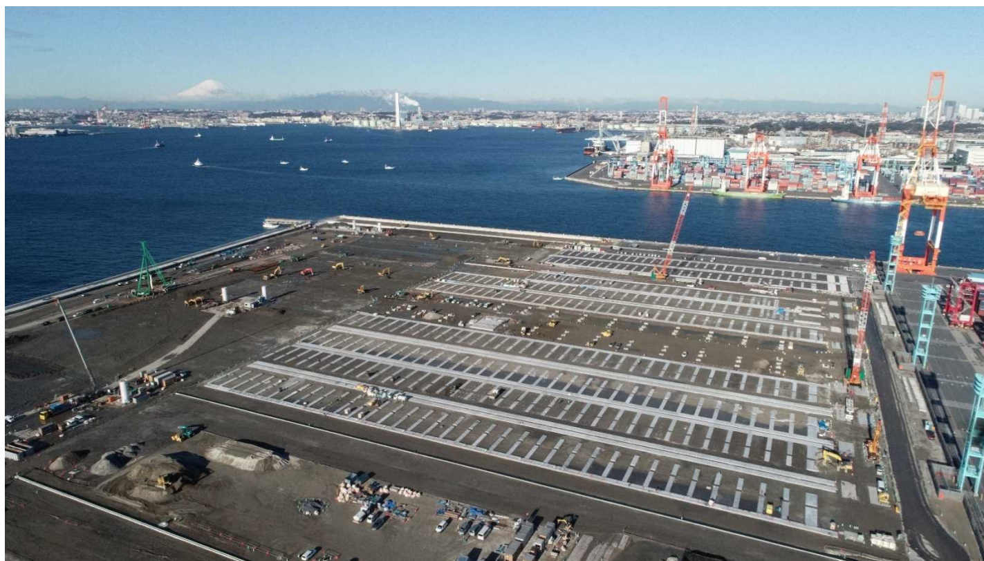
横浜港南本牧地区コンテナヤード整備【京浜港湾事務所】
