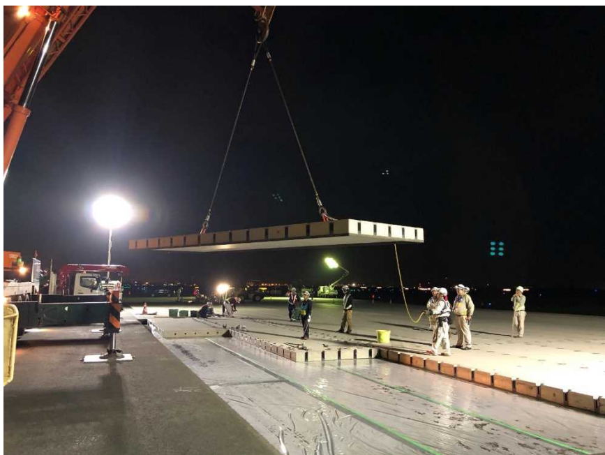
東京空港整備【東京空港整備事務所】 (左) 東側整備地区エプロン舗装PRC版敷設 (右上) 際内トンネル内 (右下) 国際線地区連絡橋ランプ部桁架設
