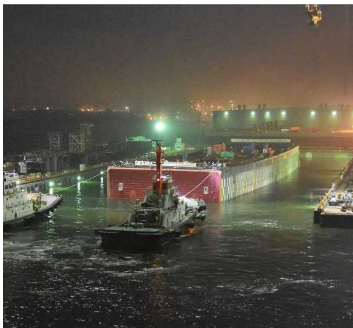
東京港南北線沈埋函（7号函）出渠【東京港湾事務所】
