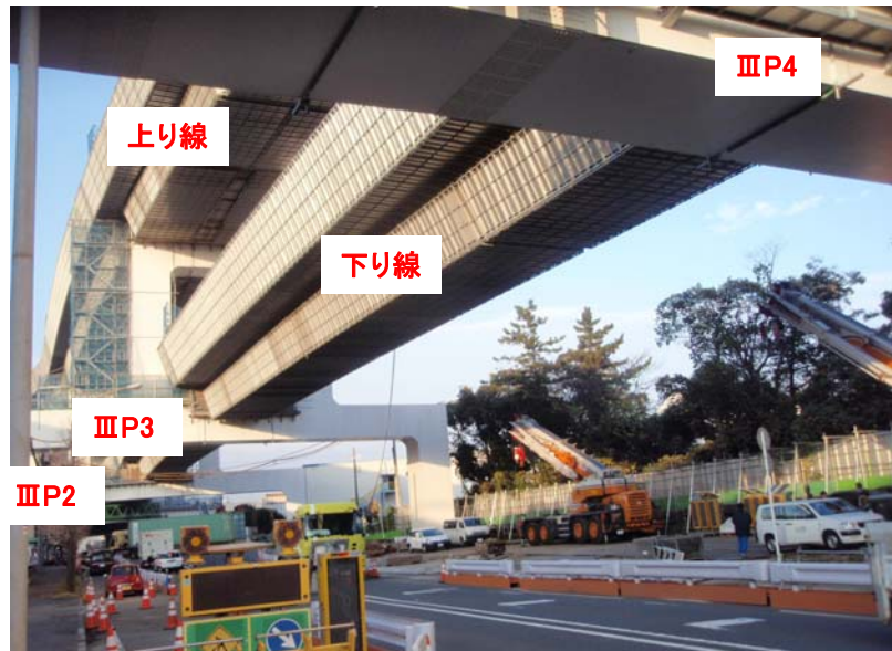
架設支保工撤去後の状況(平成27年12月中旬撮影)
