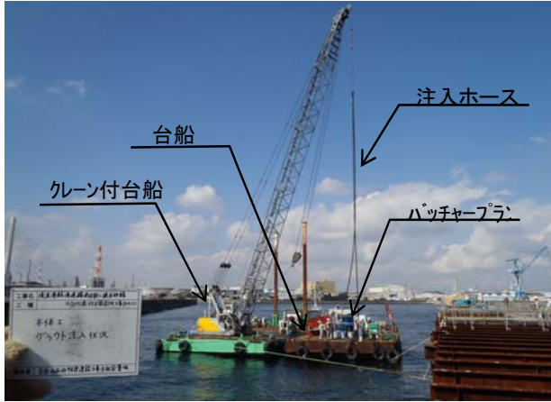
①グラウト注入状況
