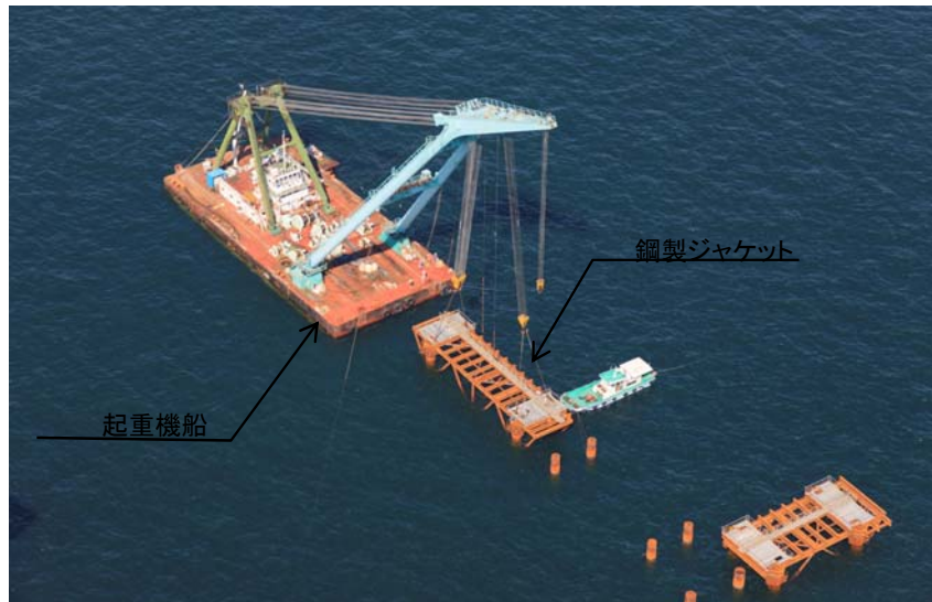
①ジャケット据付状況
