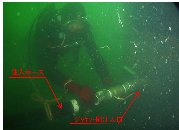
注入ホース接続状況(水中部)
