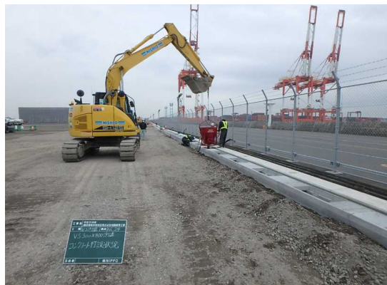
側溝工 底打ちコンクリート打設 令和2年2月
