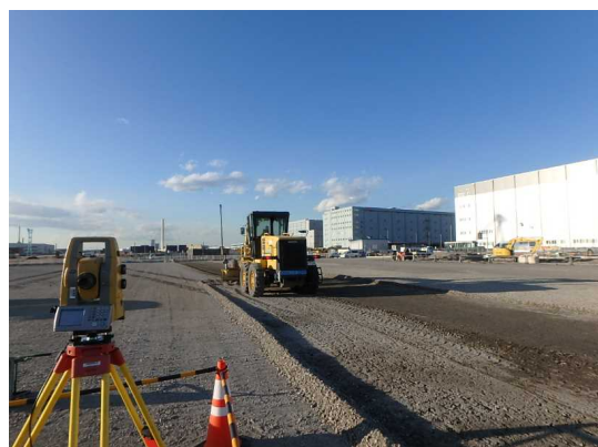
上層路盤工 仕上げ 令和2年2月
