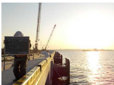
防舷材設置
