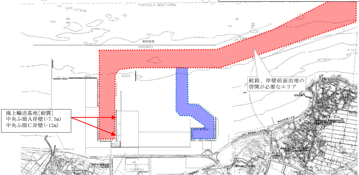
図2 茨城港地域における大規模地震時の航路啓開の考え方
