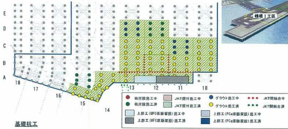
栈橋 I 工区 工事進捗平面
