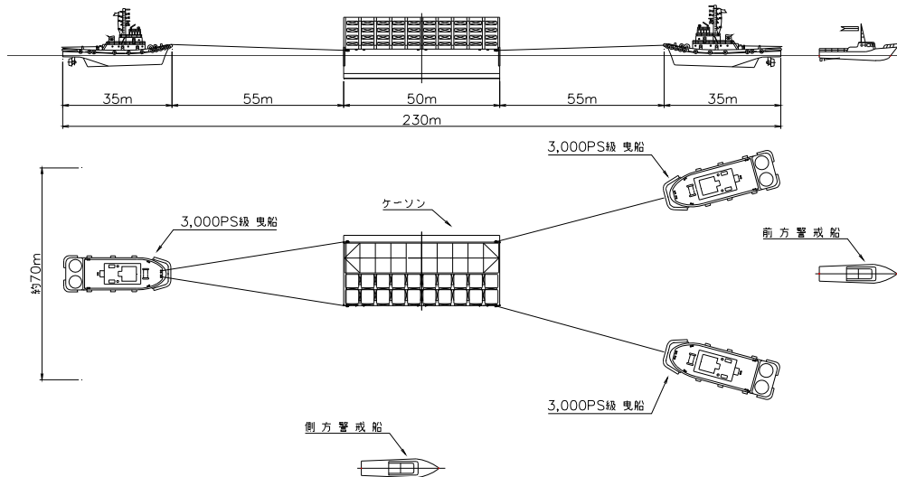
ケーソン曳航状況図(三井造船(株)千葉事業所～千葉港内一時仮置場)
