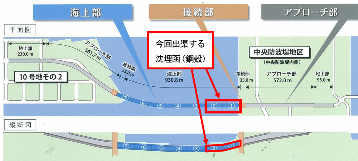
東京臨港道路南北線の概要
