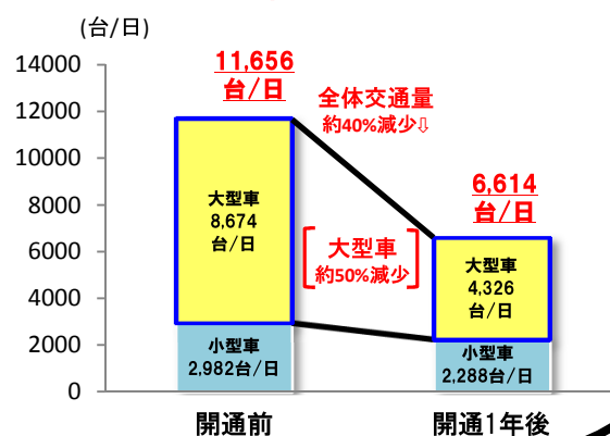
図2 南本牧大橋の交通量
