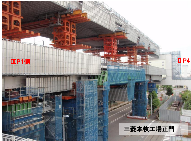
現地 平成27年6月初旬時点桁架設状況 (上り線 III P1～II P4/下り線 III P4～II P4)
