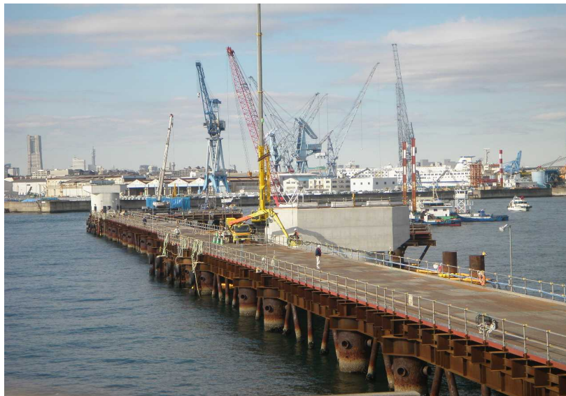
P3橋脚～P2橋脚 全 景
