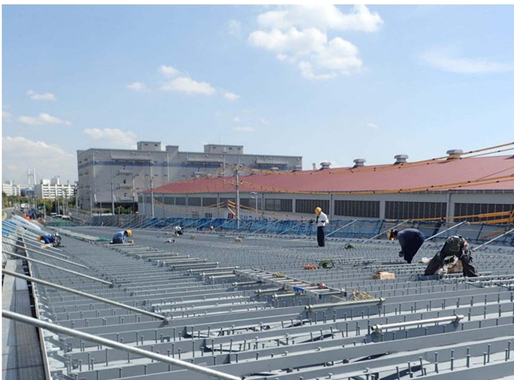
写真③ I工区 合成床版パネル架設完了
