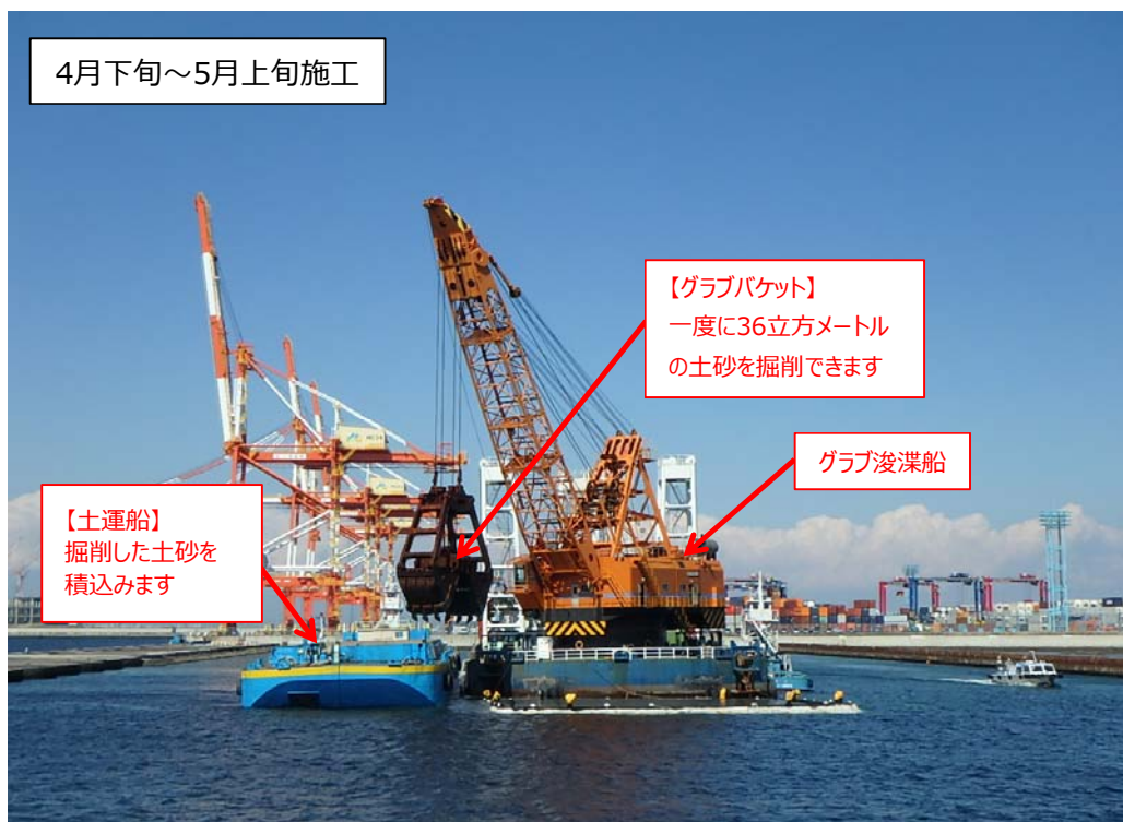
写真① 床掘工：グラブ浚渫船で海底を掘削している状況です。
