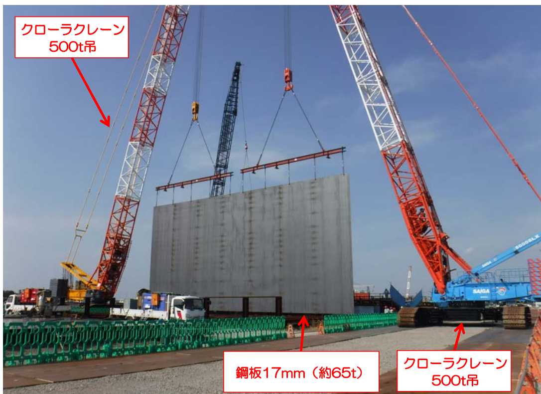
写真② 鋼板セルの鋼板（1/5分割分）に補強部材を取付ている状況です。
