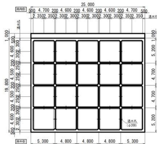
標準部平面
