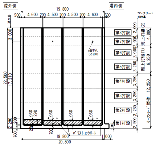
標準部断面
